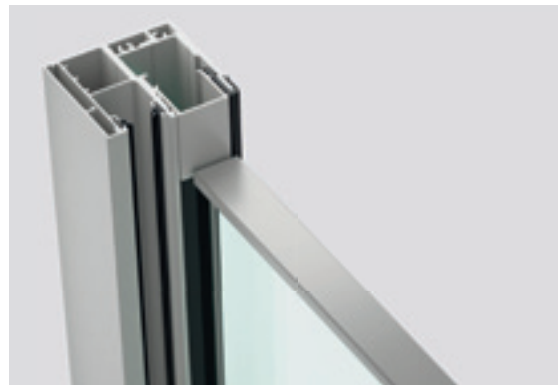
Integrierte Glas-Absturzsicherung im Vorbaurollladen
